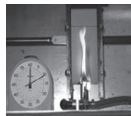
شکل ۱. تجهیزات و شیوه آزمون استاندارد EN ISO 11925-2
