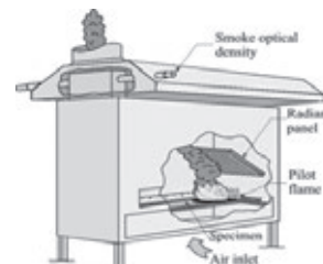
شکل ۲. تجهیزات و شیوه آزمون استاندارد EN ISO 9239-1
